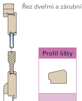
Řez dveřmi a zárubní
